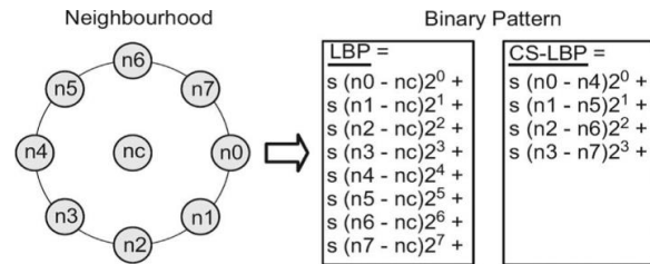
شکل ۷. ویژگی‌های الگوی دودویی محلی متقارن مرکزی و الگوی دودویی محلی برای مجاورت هشت بیکسل
