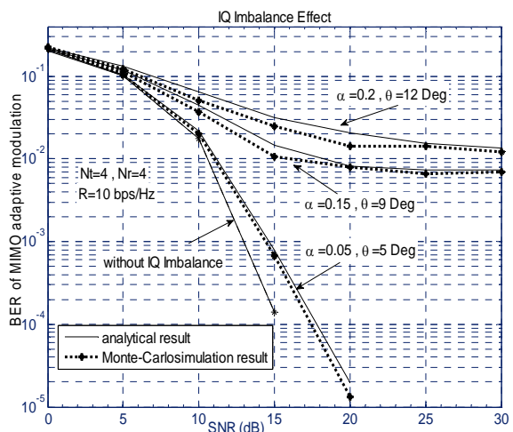
شکل ۸: احتمال خطای بیت متوسط مدولاسیون تطبیقی در سیستم‌های MIMO تحت تأثیر عدم توازن IQ به ازاء \alpha و \theta های مختلف. N_t = 4, N_r = 4 و R = 10 \text{ bps/Hz} .
