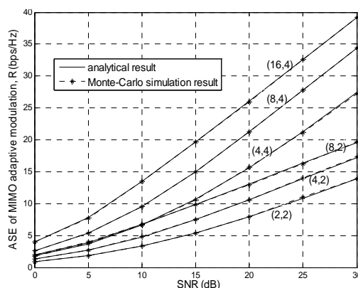
شکل ۴: بازده طیفی متوسط مدولاسیون تطبیقی در MIMO، به ازاء ۶ سیستم MIMO مختلف
